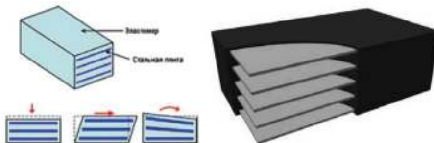
Рис 2. Опорные части из резины, усиленные стальными пластинами
